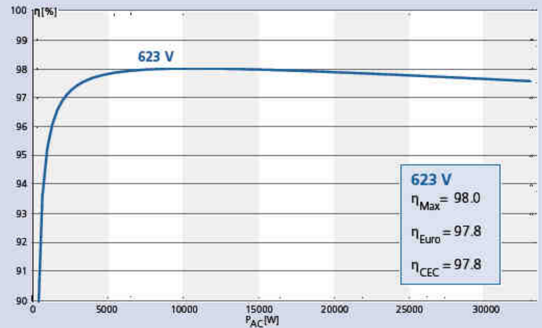
Wirkungsgradkennlinie Powador 39.0 TL3
