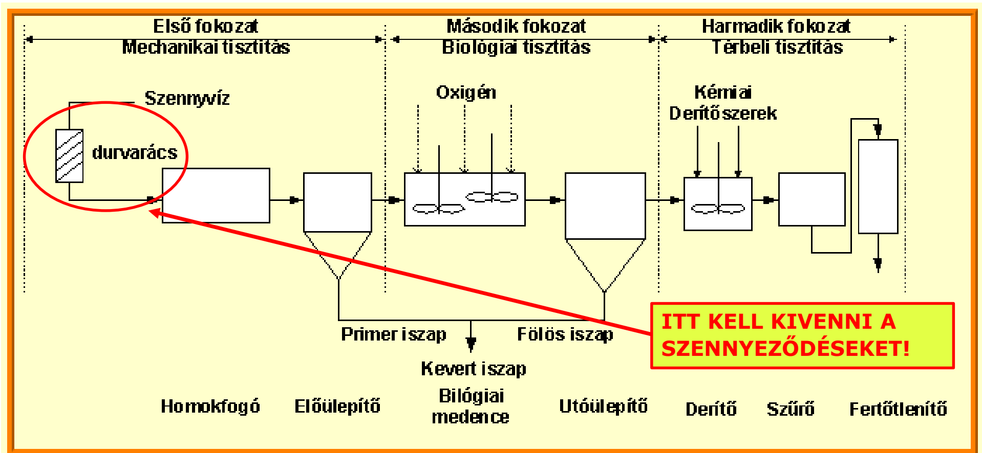
A szennyvíztisztítás általános folyamatábrája
